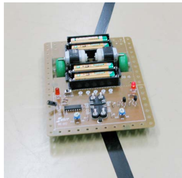
作製したライトレースカーの走行テスト
