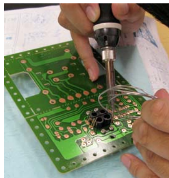
センサー基板のはんだ付け
