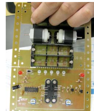
モータ部の製作
